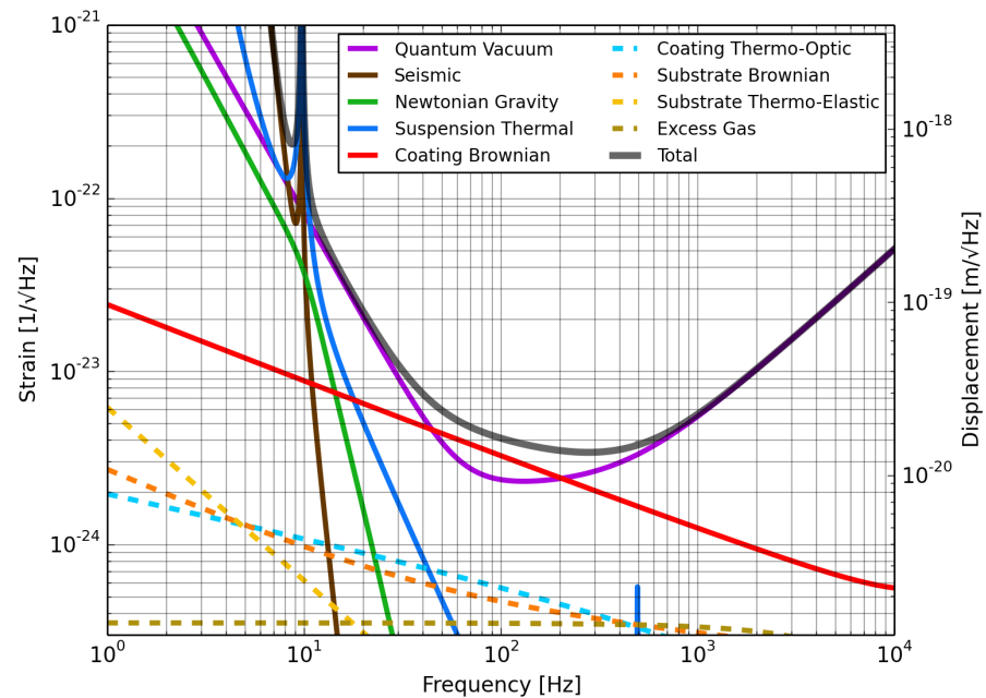
aLIGO
