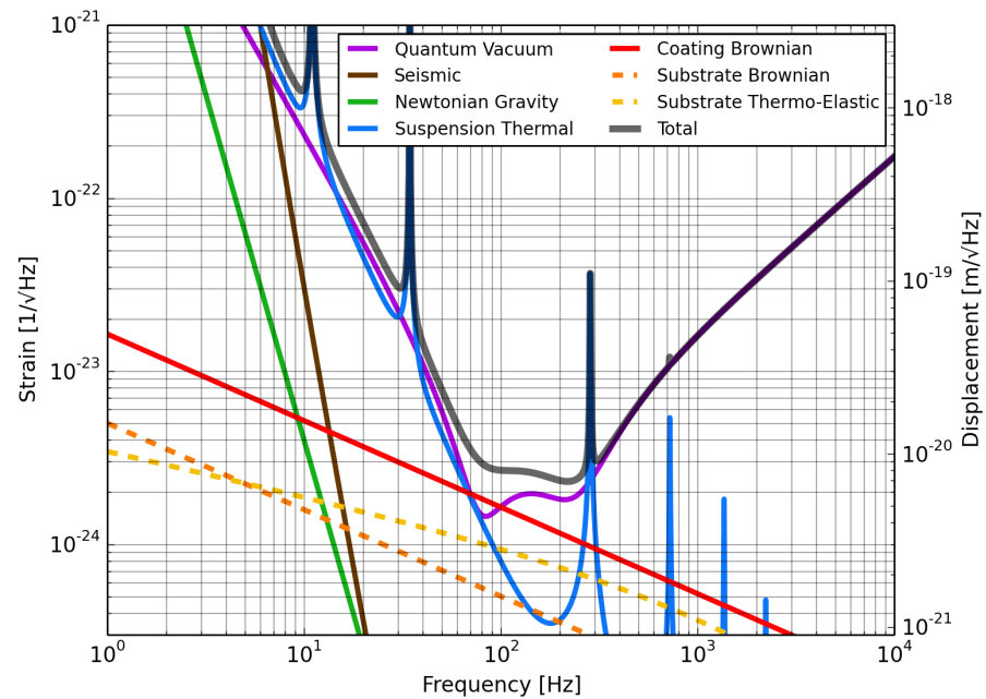
KAGRA+ (40kg)
