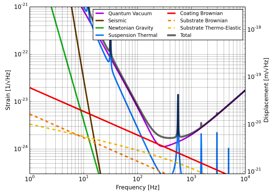
KAGRA+ (HF)
