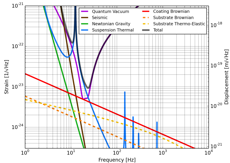
KAGRA+ (LF)
