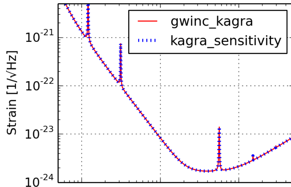
KAGRA+ (HF)
