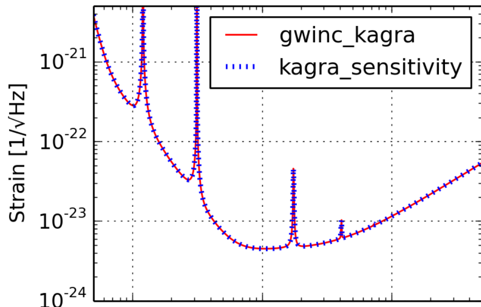
bKAGRA (BRSEhomo)
