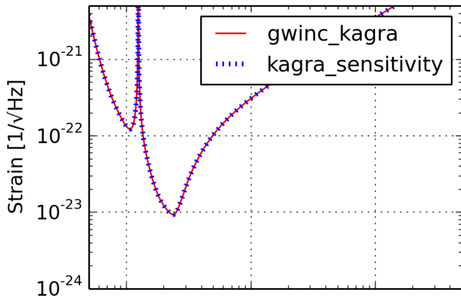
KAGRA+ (LF)
