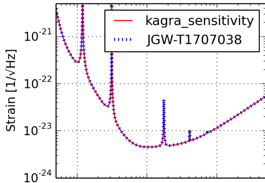
bKAGRA (BRSEhomo)
