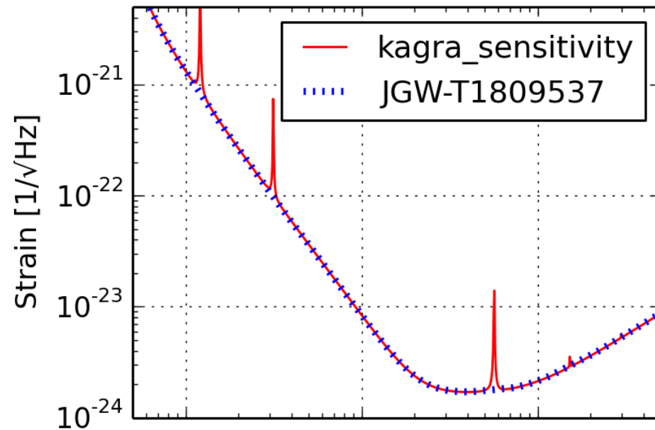
KAGRA+ (HF)
