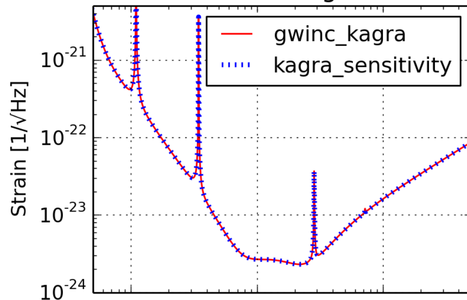
KAGRA+ (40kg)
