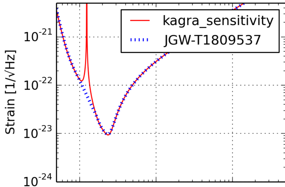
KAGRA+ (LF)
