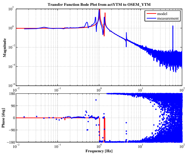
Figure 5.28: TM-OSEM (Yaw)
