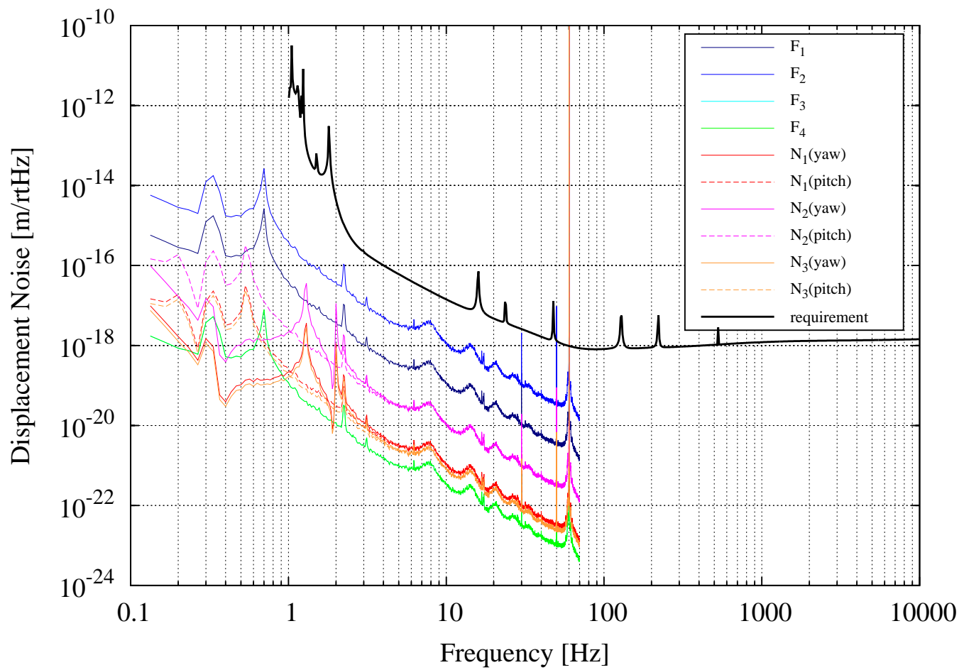
図5 BSにおける磁場雑音の計算結果。 F_1 \sim F_4, N_1 \sim N_3 の寄与をそれぞれ異なる色で示した( F_3 と F_4 は重なっている)。 N_1 \sim N_3 に関しては、更にそれぞれ鏡のyaw,pitchを通した寄与があるので、それらを実線(yaw)と鎖線(pitch)で表している。
