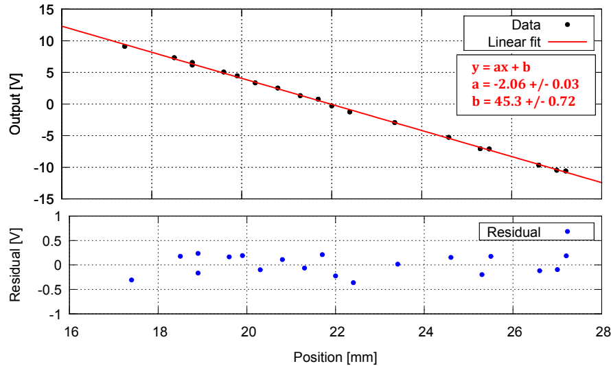
Figure 5.7: LVDT のキャリブレーション結果
