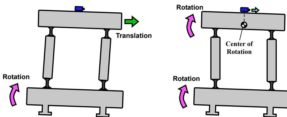
Figure 5.20: ベースの傾きからトップステージ上の水平加速度計へのカップリング
