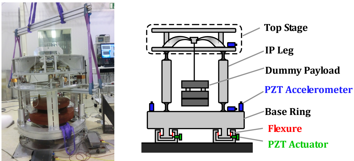
Figure 5.23: GAS フィルターの伝達関数測定のセットアップ
