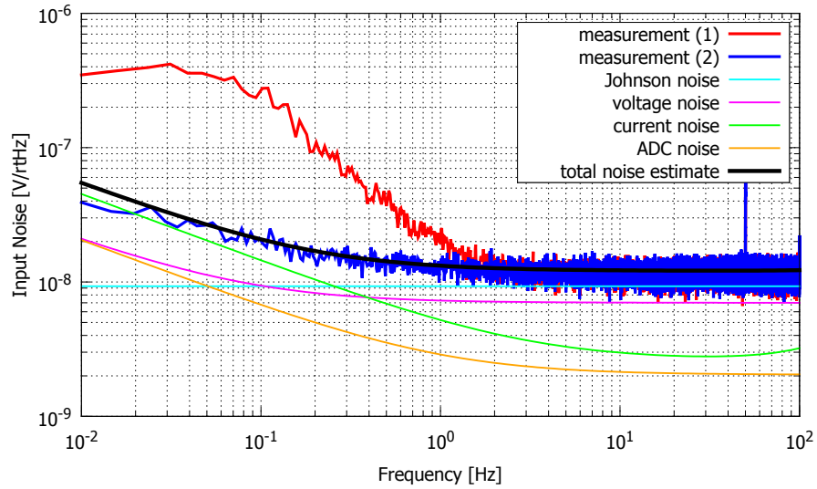
Figure 5.11: プリアンプの入力換算雑音。赤線と青線が実測データ、その他の細線が推定される雑音源のスペクトルを表し、黒い太線がその総和を表す。
