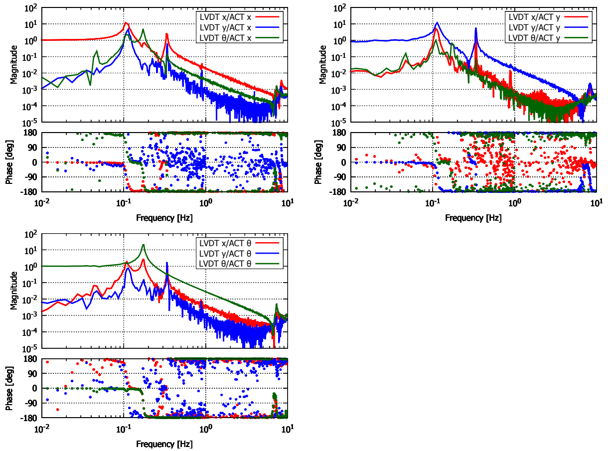
Figure 5.15: 対角化されたアクチュエータから LVDT で測定されたステージ変位への伝達関数
