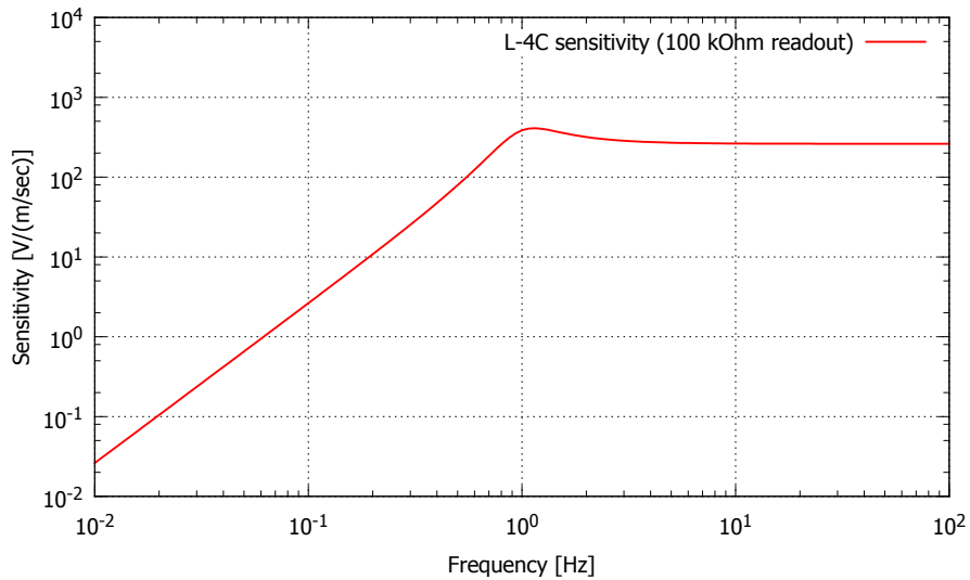
Figure 5.9: L-4C の地面振動に対する周波数応答
