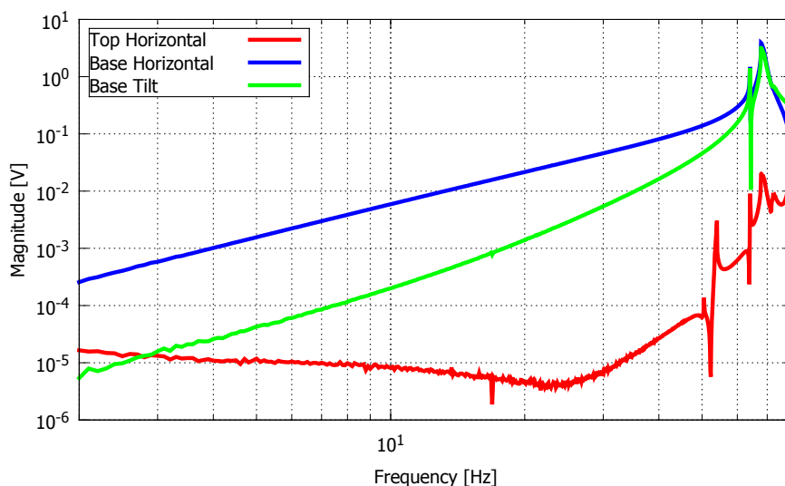
Figure 5.18: 加速度計の周波数ごとの出力電圧振幅
