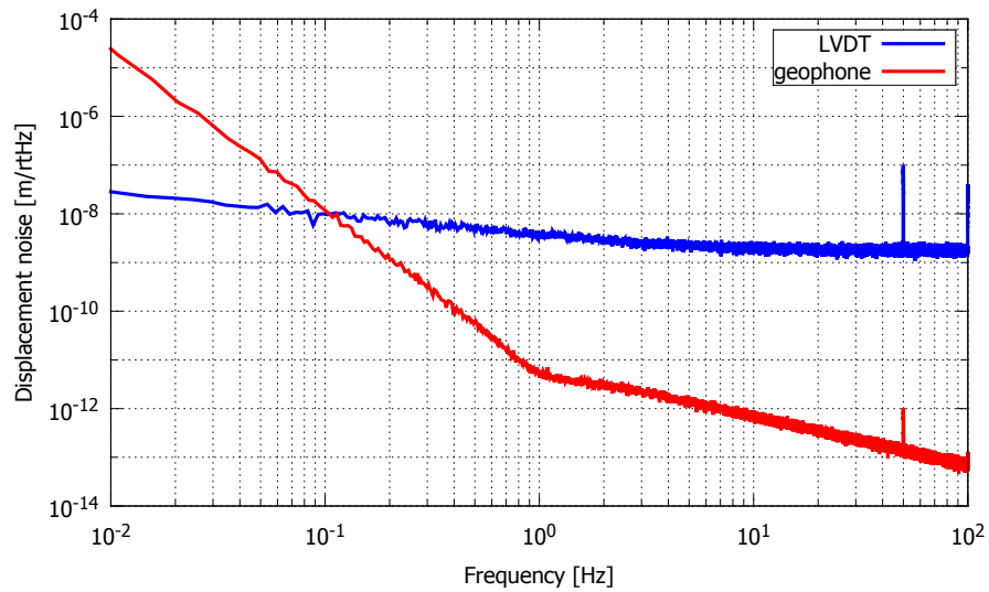
Figure 5.12: Geophone と LVDT の変位雑音レベルの比較
