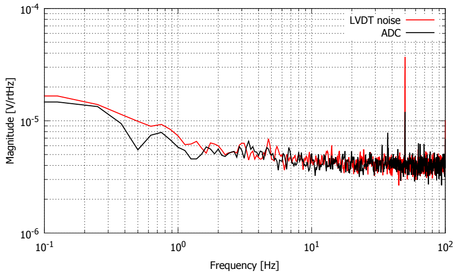
Figure 5.8: LVDT の雑音スペクトルと ADC の雑音の比較
