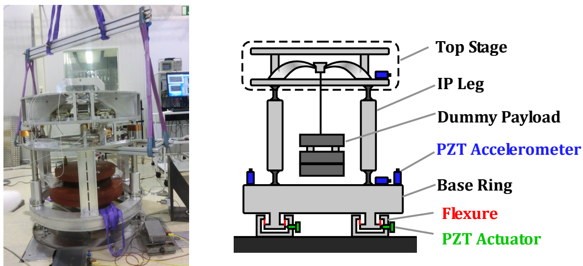
Figure 5.17: multi-SAS 用倒立振り子の伝達関数測定のためのセットアップ
