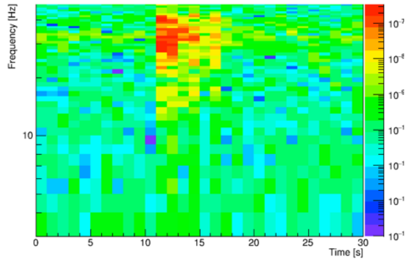
K1:PEM-EX_ACC_NO2_X_FLOOR
