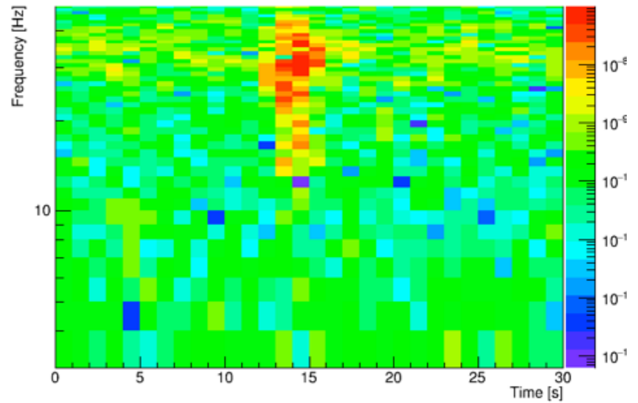
K1:PEM-EX_ACC_NO2_X_FLOOR
