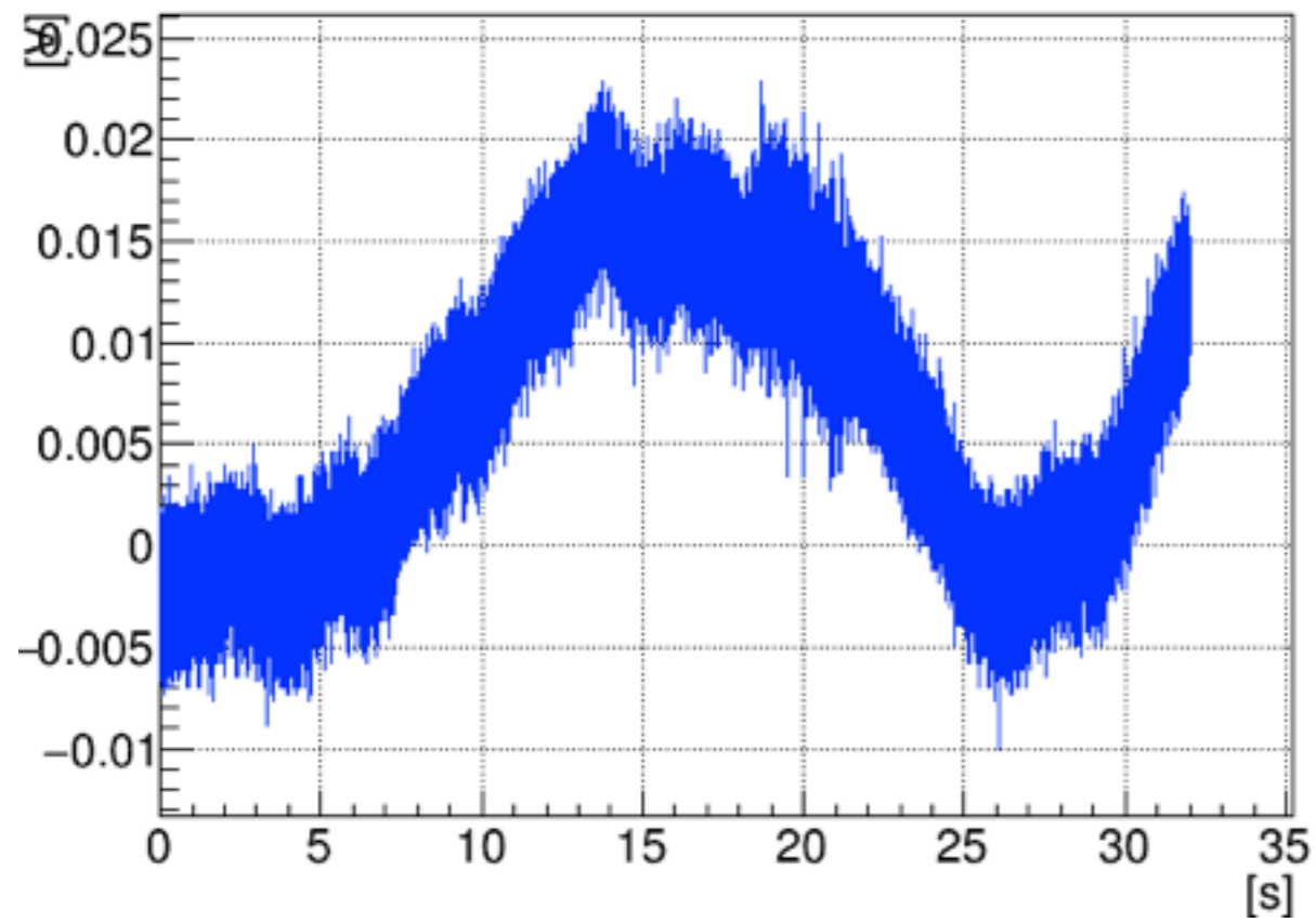
K1:PEM-EX_ACC_NO2_X_FLOOR
