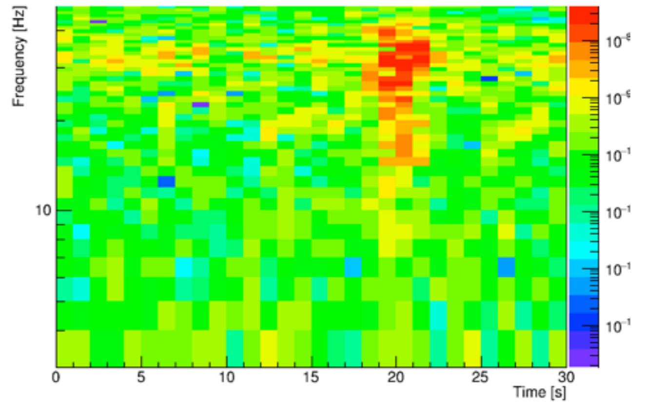
K1:PEM-EX_ACC_NO2_X_FLOOR
