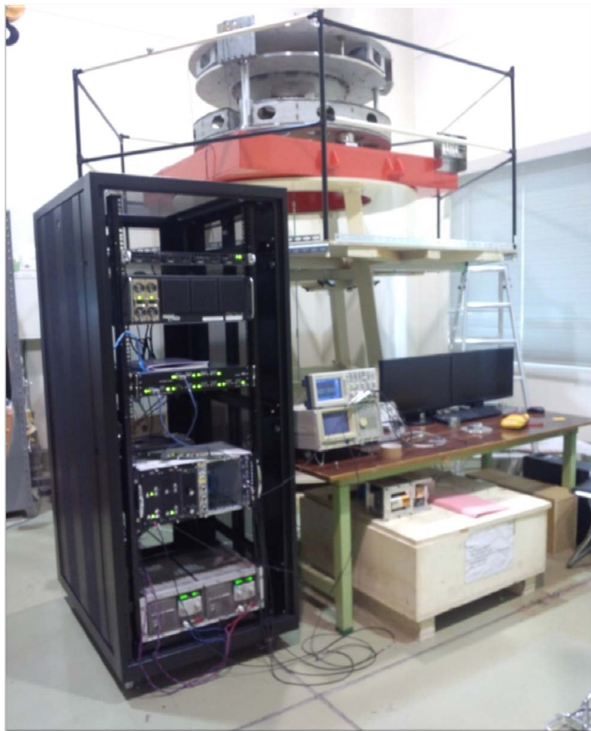
Pre-Isolatorのプロトタイプテスト(@柏)
