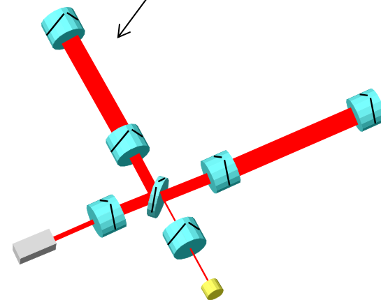
Resonant Sideband Extraction干涉計 (第2世代技術)
