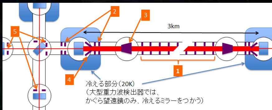
KAGRAハッフル構成図
