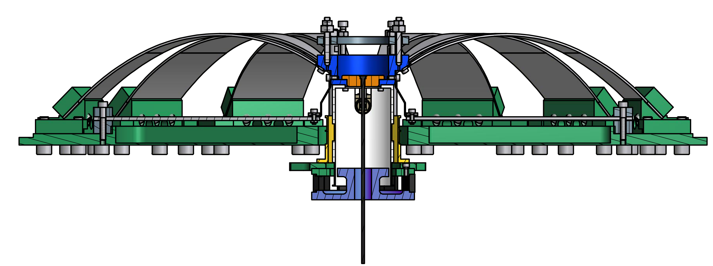
B-B ( 1 : 2.5 )
