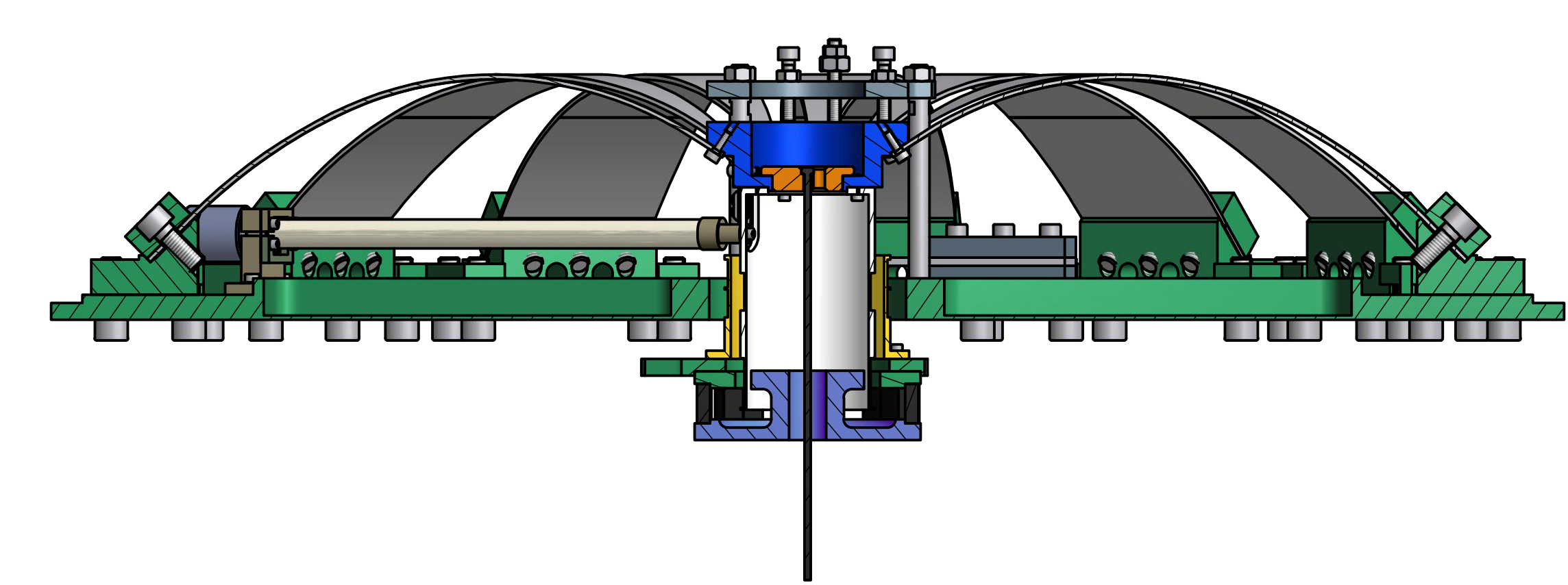
C-C ( 1 : 2.5 )
