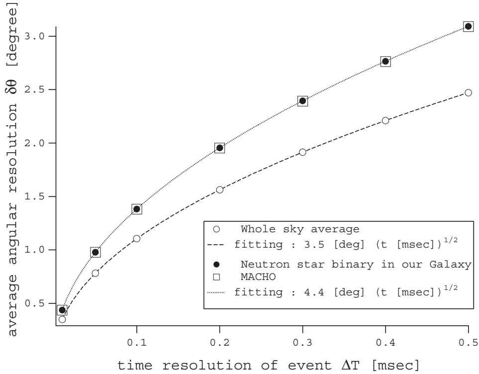
図 18.10: 重力波源方向の決定精度
