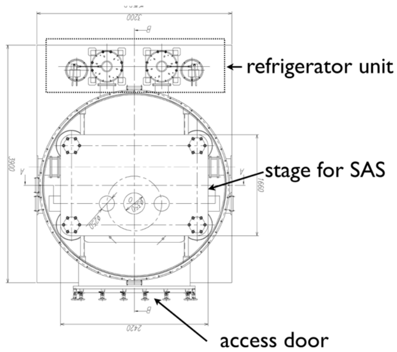
図 10.9: クライオスタット上面図。
