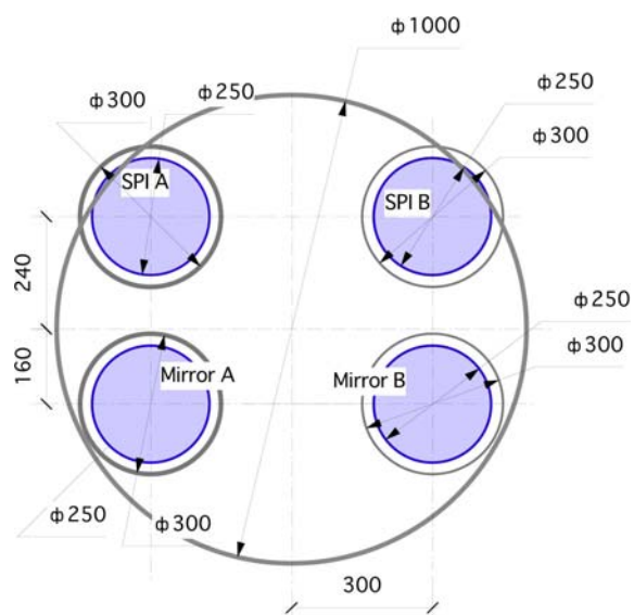
図 10.3: 鏡配置図。4 本のレーザービームが直径 1000 mm、長さ 3 km の真空パイプを共有している。二干渉計間隔は 600 mm、鏡直径は 250 mm、低温真空パイプの直径は 300 mm、低温真空パイプ内の輻射シールドの直径は 250 mm である。振り子最終段の長さは 400 mm。直径 1000 mm の真空パイプから、変換フランジ、ゲートバルブを介して、4 本の各ビーム用の真空パイプが取り付けられる。
