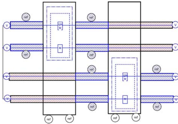
図 10.4: 干渉計 A、B 用低温システム配置図。「V」はゲートバルブ、「ref」は冷凍機、「SPIM」は SPI 用鏡、「M」は主干渉計用鏡を示す。「SPIM」、「M」が二重の点線に囲まれているのは、クライオスタット内部の輻射シールドに囲われた低温部につり下げられることを示す。青い斜線部が低温真空パイプ、赤い斜線部が常温真空パイプを示す。クライオスタット内を貫通する常温真空パイプはそのクライオスタットとは独立の真空を持つ。
