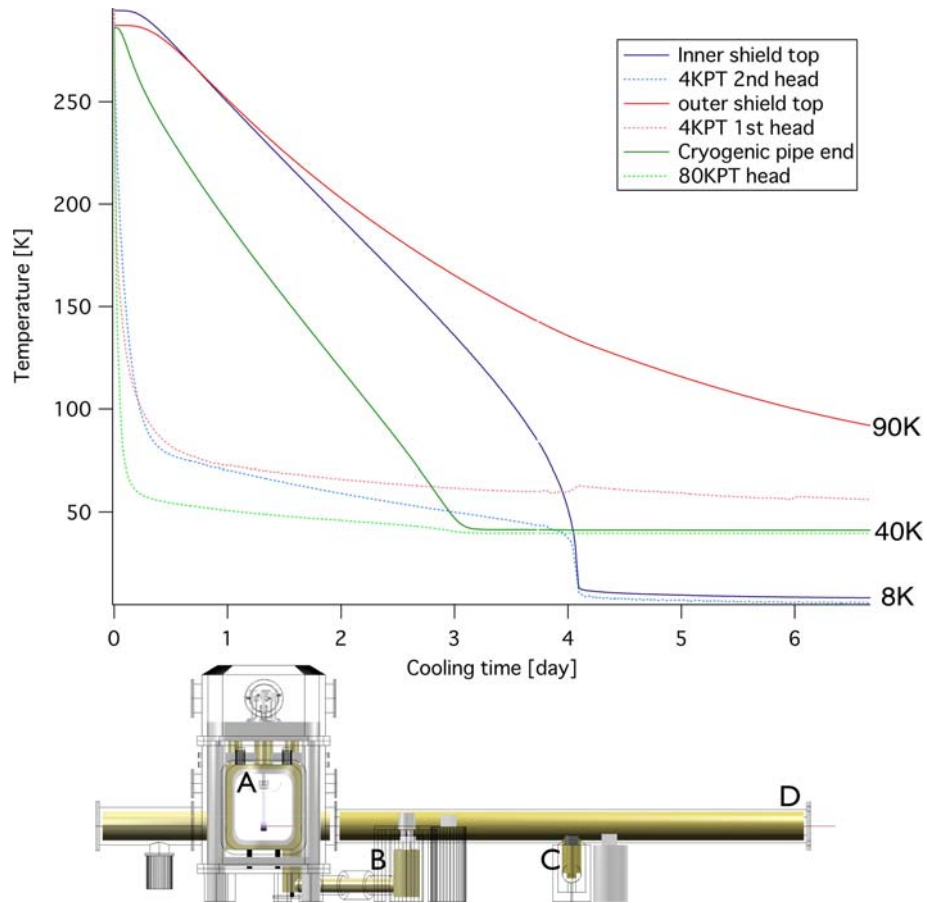
図 10.11: CLIO 冷却試験結果。下図は冷却システムの内面図を示す。「Inner shield top」、「outer shield top」は各シールドの図中「A」点、「4KPT 1st head」、「4KPT 2nd head」は「B」点にあるクライオスタット用冷凍機、「80KPT head」は「C」点にある、低温真空パイプ用冷凍機、「Cryogenic pipe end」は「D」点が相当する。到達温度は仕様を満たしている。
