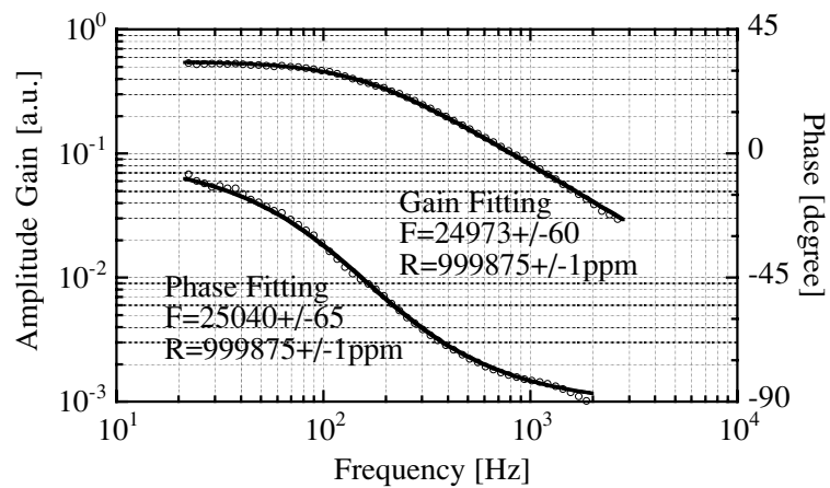
図 8.13: 基線長 20m のレーザー干渉計で測定した共振器の周波数応答．これよりフィネスは約 25,000，反射率 99.9875%，損失 28ppm となる．
