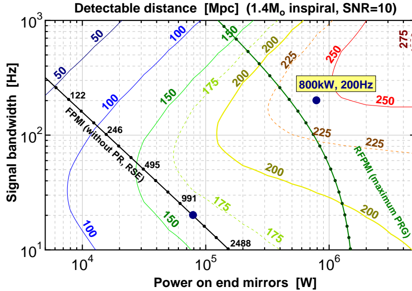
図 4.4: 1.4M_{\odot} - 1.4M_{\odot} の連星合体からの重力波を \text{SNR}=10 で検出できる距離．重力波源の方向と偏波成分としては, 干渉計の感度が最も高くなるものを仮定している．従って, 全平均すると, この距離は 1/\sqrt{5} になる．横軸は, 干渉計内光強度 (両腕共振器内光強度の和) で, 縦軸が信号帯域幅となっている．干渉計内光強度 800 kW, 信号帯域幅 200 Hz の点が LCGT のデザイン値を表す．このとき, 240 Mpc の現象まで捉えることができる．
