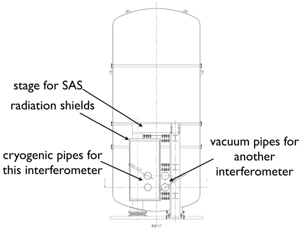
図 10.7: クライオスタット内面図。
