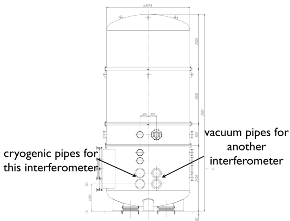
図 10.6: クライオスタット前面図。直径約 3000 mm、高さ 7200 mm。主干渉計用ビーム高さは床上 1000 mm、SPI 用ビーム高さは床上 1400 mm。
