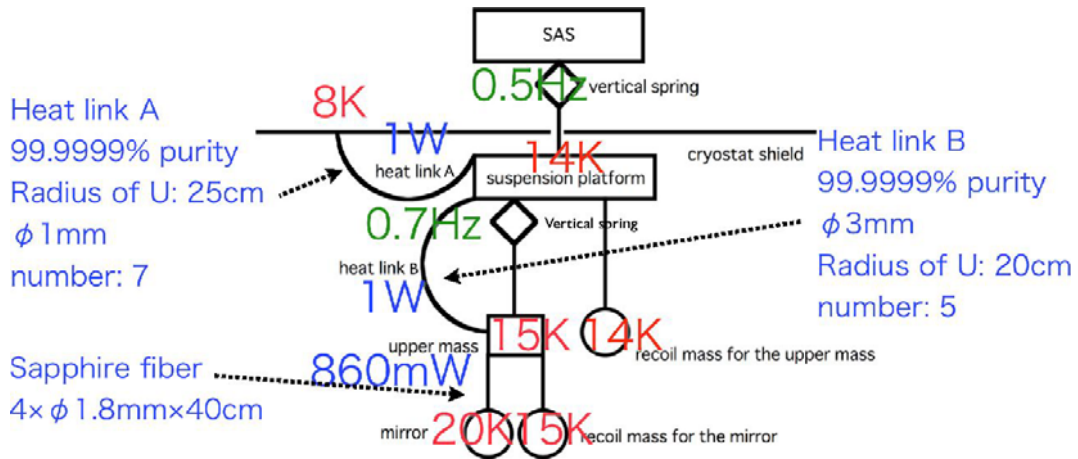
図 10.15: ヒートリンクデザイン。鏡で発生した熱は直径 1.8 mm、長さ 400 mm の 4 本のサファイアファイバーを伝ってアップパーマスへ流れる。サファイアファイバーを用いることで Q 値の高い振り子 ( Q = 10^8 ) [4] と高い熱伝導 [7][8] の両方を実現できる。予想の 3 倍にあたる 860 mW の発熱がニアミラー中にあっても鏡の温度を 20 K が達成できるように設計されている。アップパーマスの上流には「C」または「U」字型のヒートリンクが張られている。このような形で張るのは、ヒートリンクの剛性を下げ、振動の伝達を低減するためである。このヒートリンクは高純度アルミニウム線 (純度 99.9999%) を用いる。ここでも予想の約 3 倍の 1 W の熱が流せるように設計されている。
