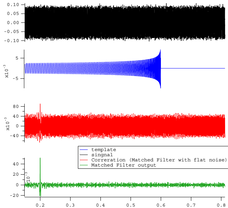
図 18.7: 相関計算例 (チャープ、雑音あり)
