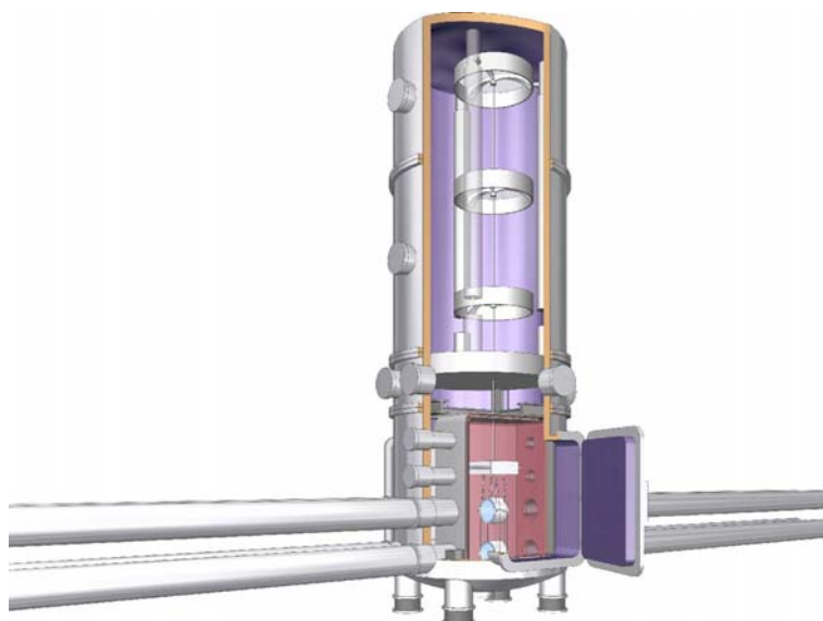
図 10.2: LCGT 用低温システムイメージ
