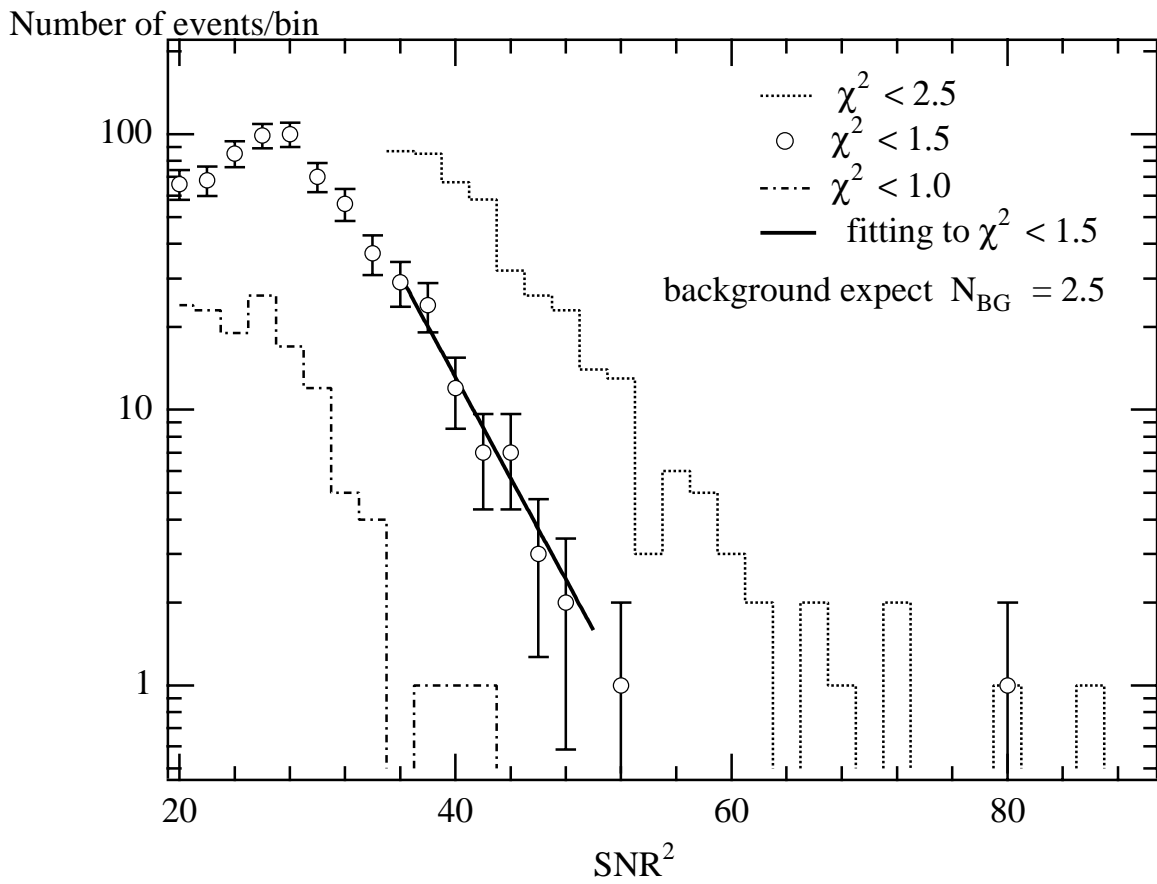
図 18.9: TAMA DT2 でのインスパイラル探索
