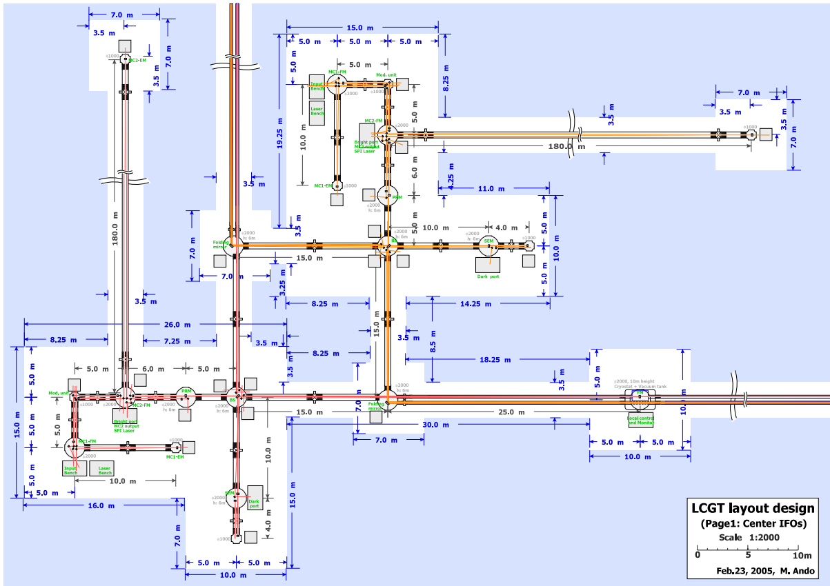
図 D.2: 神岡地下に設置される LCGT の中央真空槽室近辺の配置図。独立な 2 基のレーザー干渉計のそれぞれの光ビームは 1 本の真空ダクトの中を共通に通すが、ビームスプリッターや入射光学系は別々に独立した真空槽群に収める必要があるため、この配置図にあるようにそれぞれ 2 組の入射光学系に対応したトンネルが作られることとなる。
