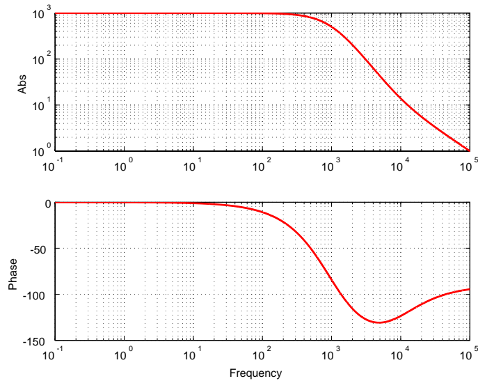
図 7.15: レーザー強度安定化システムのボード線図
