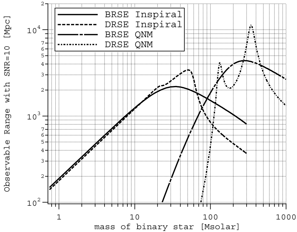
図 18.4: SNR = 10 で観測できる範囲
