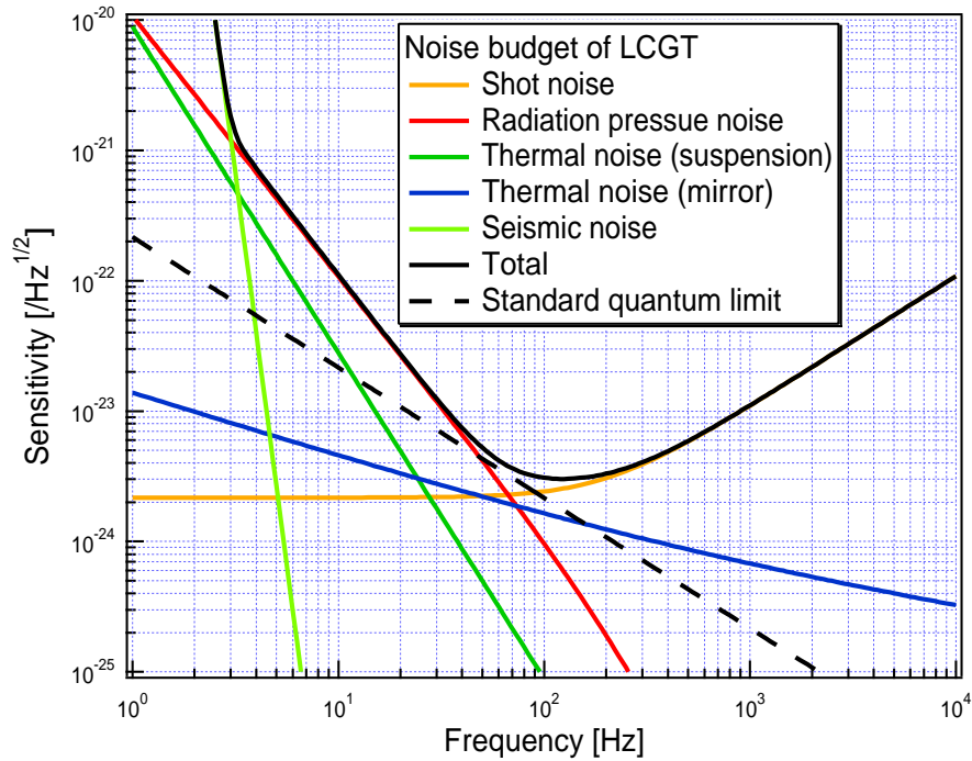
図 3.1: LCGT 計画の目標感度 : 干渉計の原理的な雑音である optical readout noise (shot noise と radiation pressure noise からなる) と thermal noise と seismic noise を示した。これらの総和 (total) が LCGT 計画の目標感度になる。ほぼ全ての帯域で optical readout noise で目標感度は決まっている。optical readout noise は不確定性原理に対応する standard quantum limit より小さくなることはないが、LCGT 計画の目標感度はその standard quantum limit に接している。
