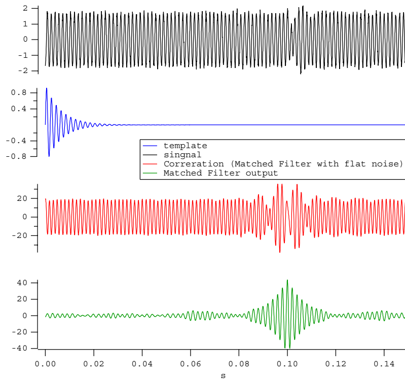
図 18.8: 相関計算例 (リングダウン、雑音あり)
