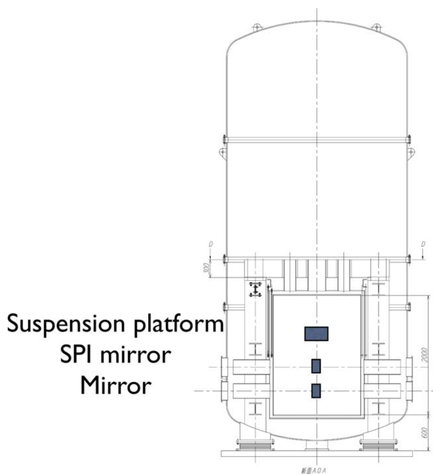
図 10.8: クライオスタット側面図。
