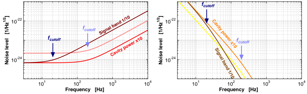
図 4.3: 量子雑音のスペクトル．分散雑音 (左), 輻射圧雑音 (右) のそれぞれについて, 干渉計内の光強度 (cavity power) と信号帯域幅 ( f_{\text{cutoff}} ) を変化させた時の様子もプロットされている．
