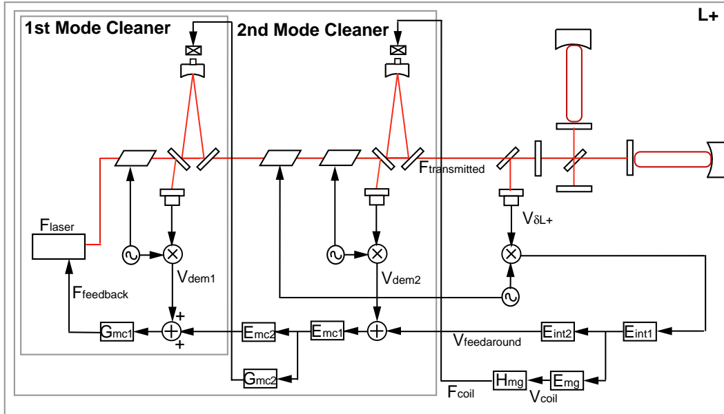
図 7.3: LCGT のサーボポロジ-: レーザ-周波数安定化に必要な変調と制御ル-ブのみを表している。
