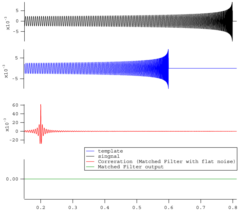
図 18.5: 相関計算例 (チャープ、雑音なし)
