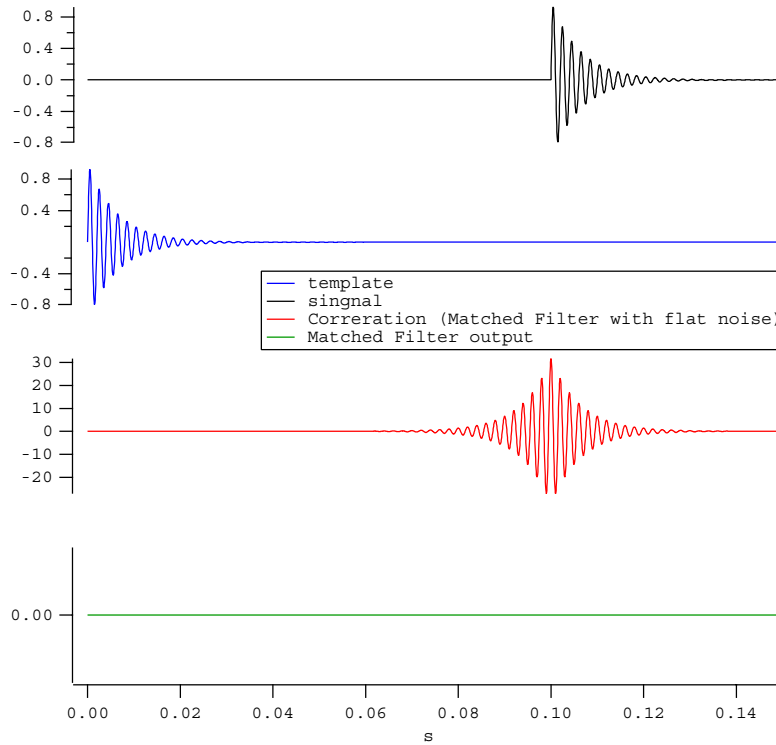
図 18.6: 相関計算例 (リングダウン、雑音なし)
